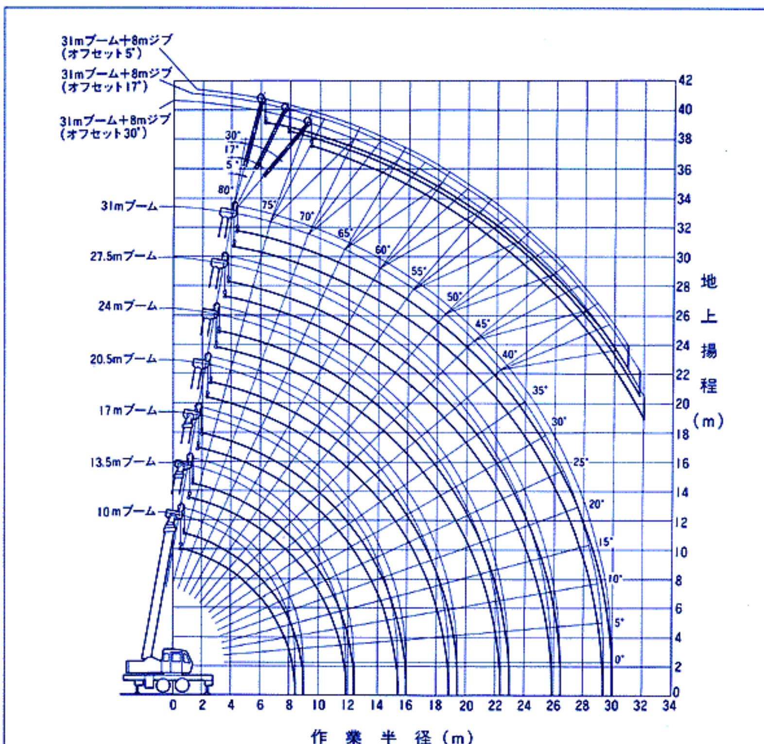
■ 作業範囲図
